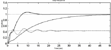
Fig. 6. c, Table II, K_p = 0.20
