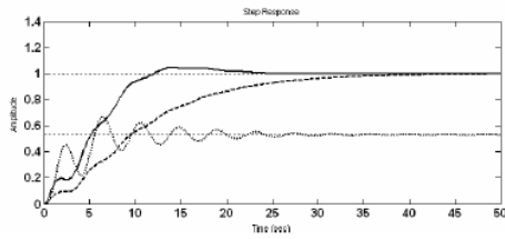
Fig. 6. b, Table II, K_p = 0.09
