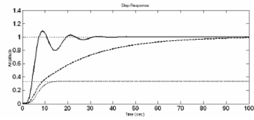
Fig. 5 c for Table I, S. No. 3
