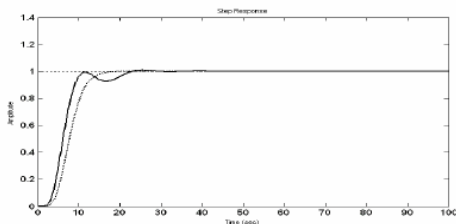
Fig. 5. a for Table I, S. No. 1
